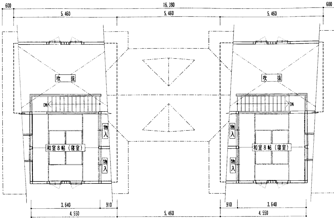
コテージ No 2
