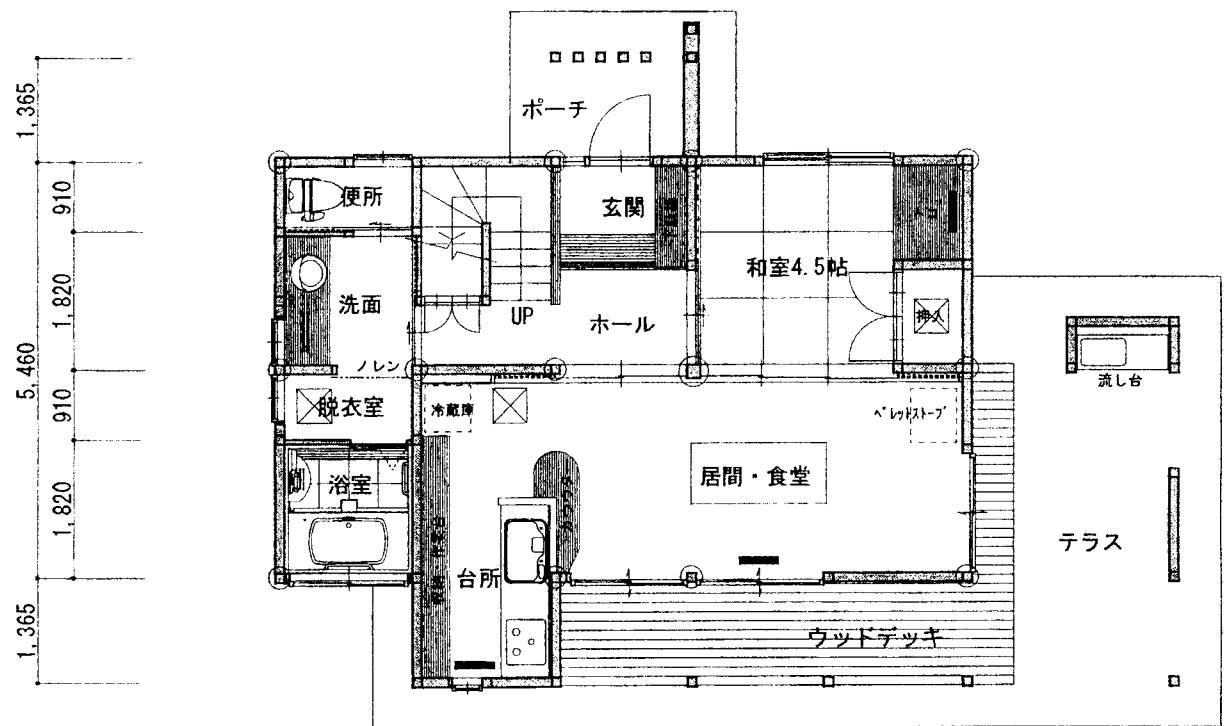
コテージ No.14
